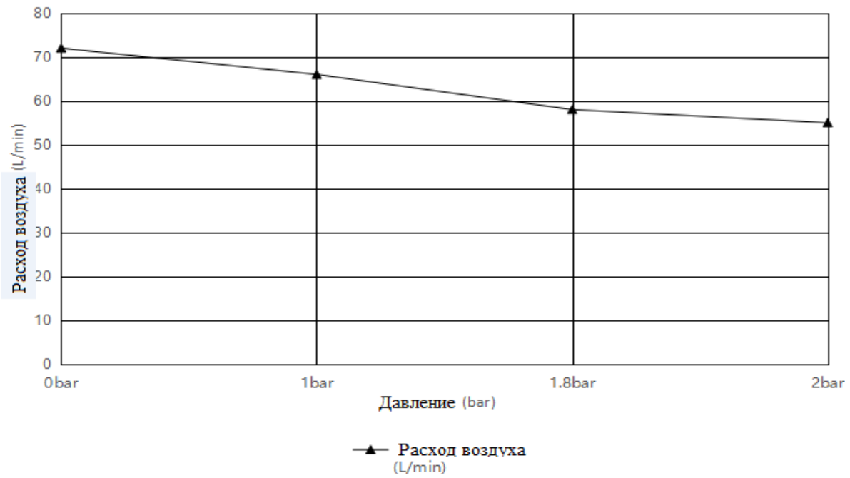
HC280A График производительности
