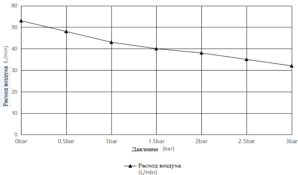
НС100А График производительности
