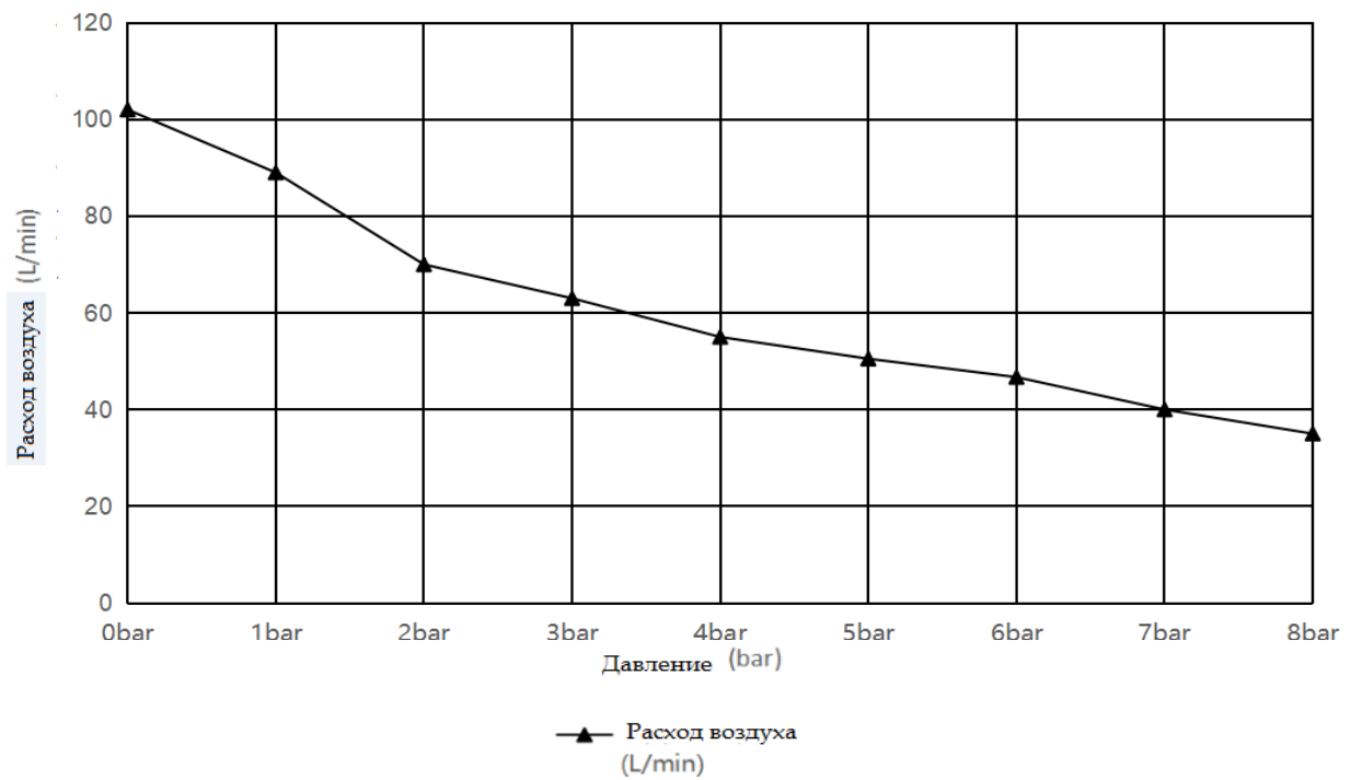
HC550A График производительности
